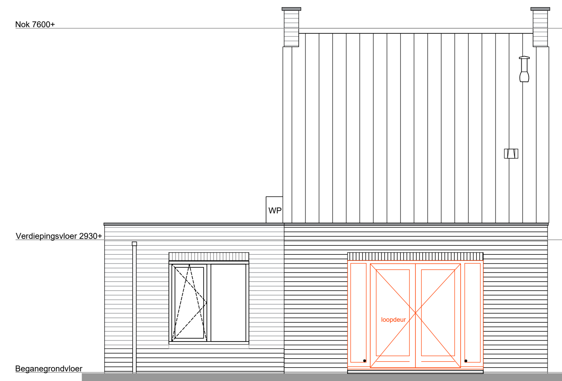
Optie B20 openslaande deuren + Optie B03BD - B04BD uitbouw woonkamer 1,2m en 2,4m
