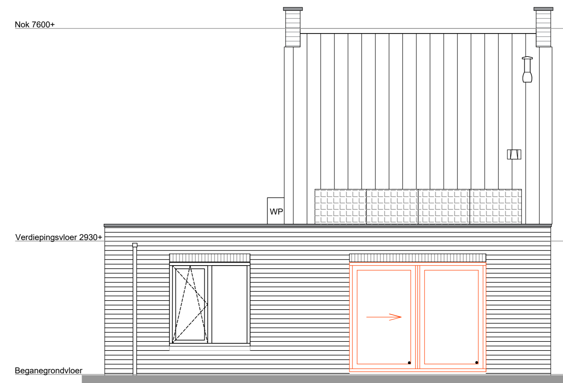
Optie B21 schuifpui + Optie B08BD uitbouw 2,4m over woningbreedte
