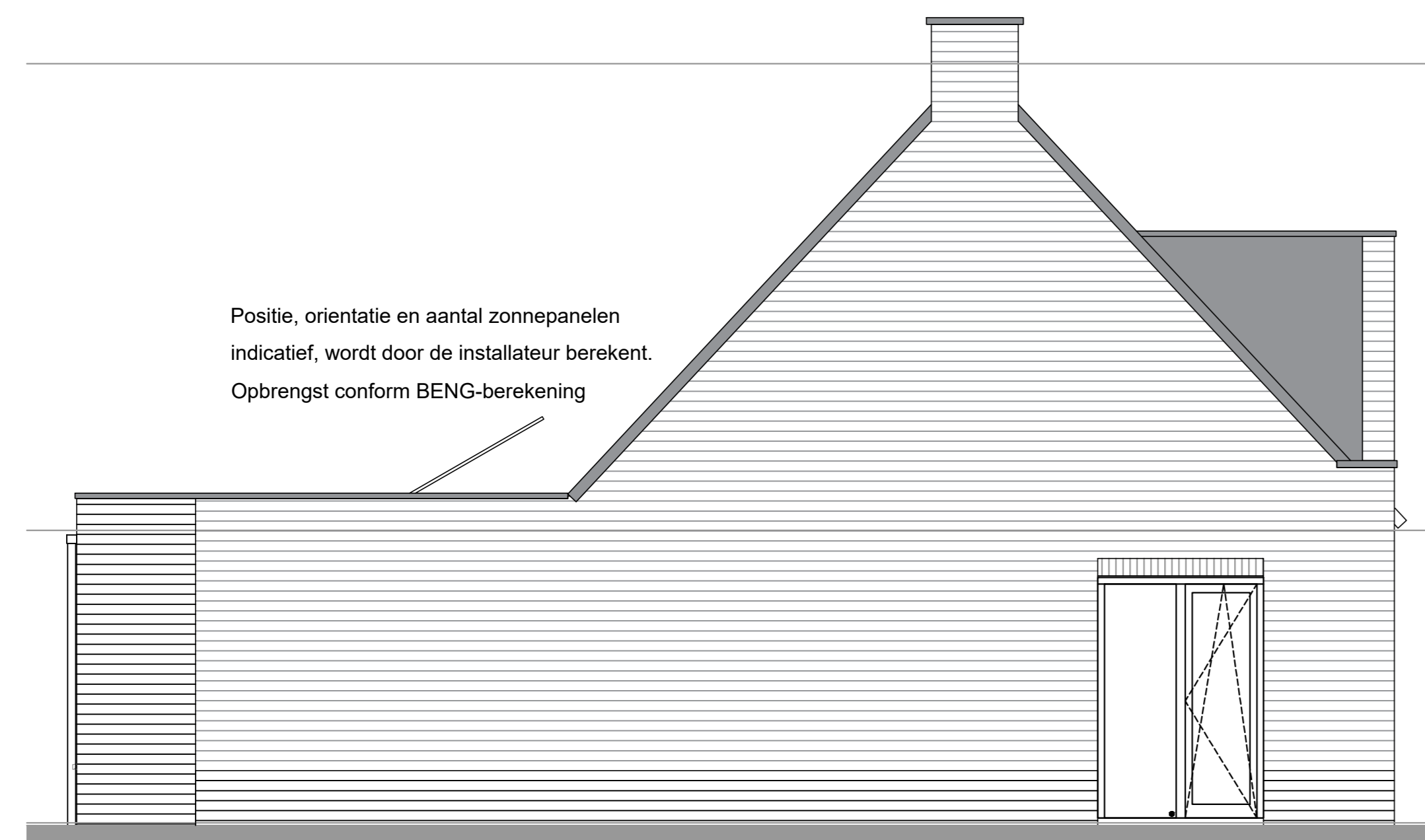
Optie B03BD - B07BD uitbouw 1,2m
