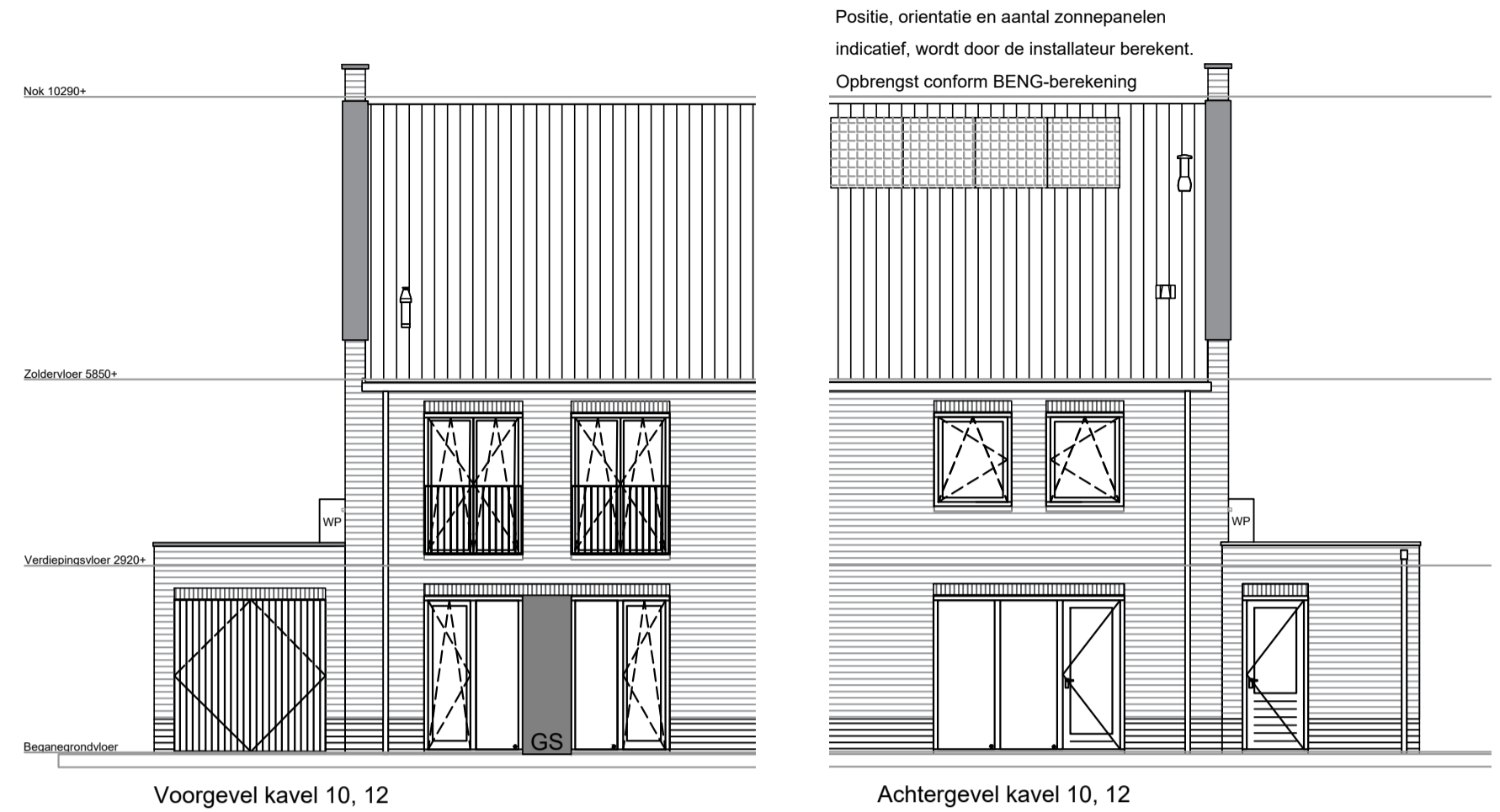
Voorgevel kavel 10, 12
