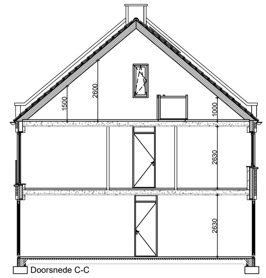
Doorsnede C-C
