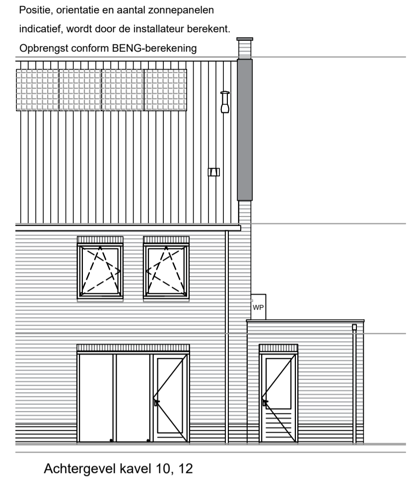
Achtergevel kavel 10, 12
